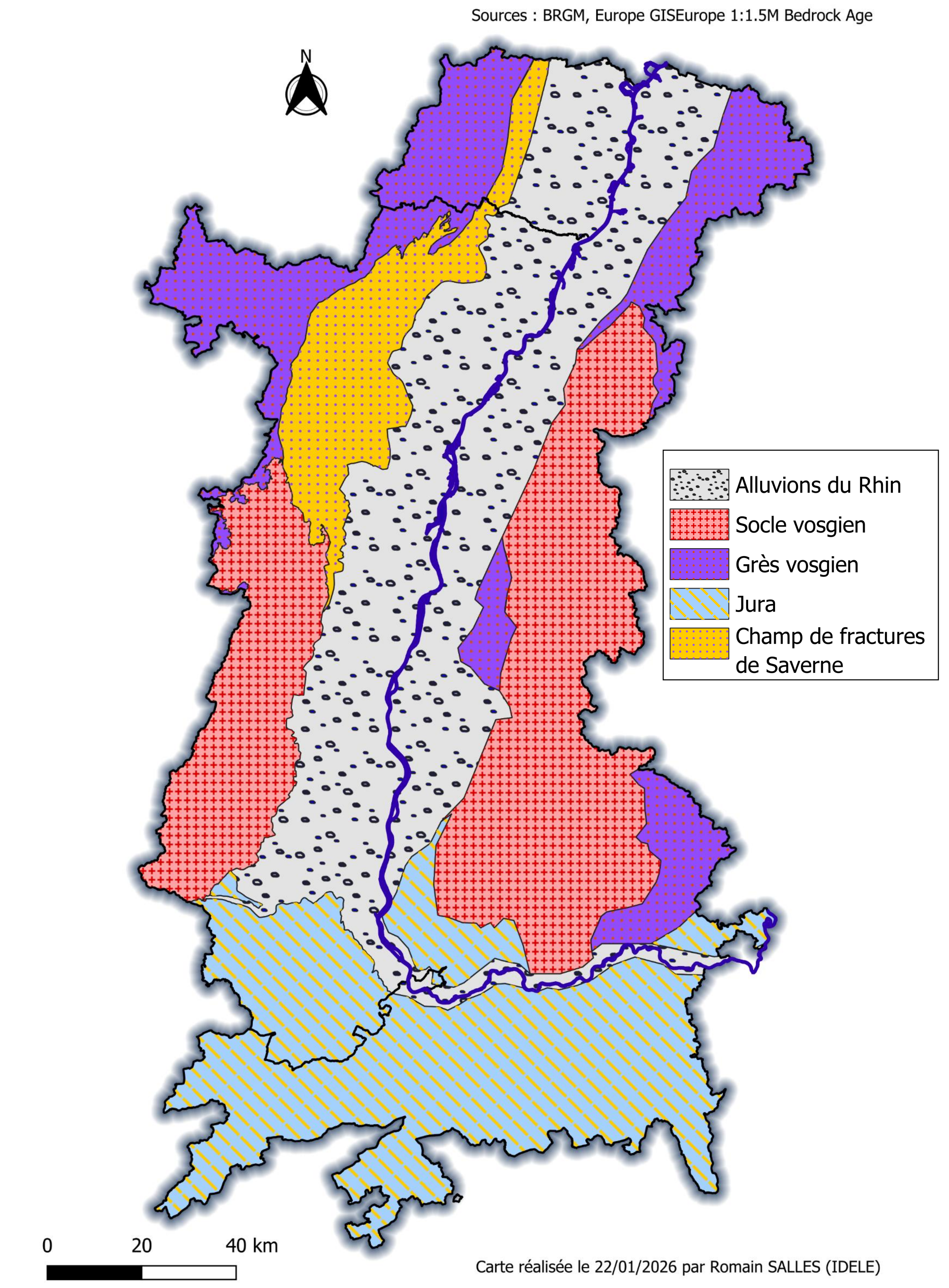
Carte géologique simplifiée
