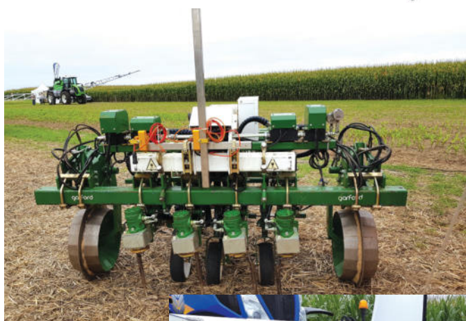
Bineuse guidée par caméra Garford
